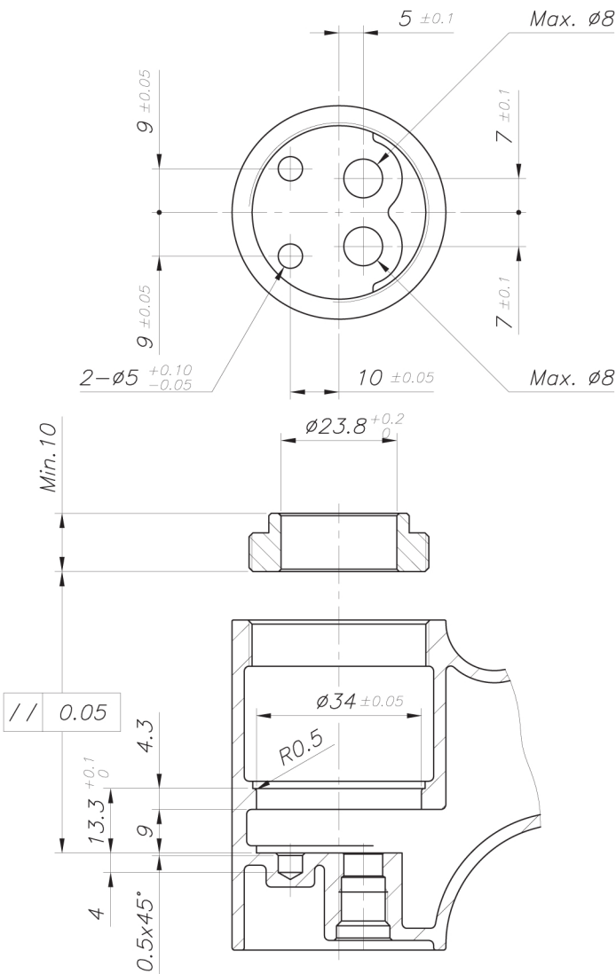
TPS35AD-1,2
